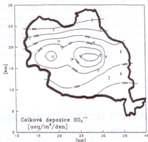
Celková atmosférická depozice v Jizerských horách patří ke zcela nejvyšším v horských oblastech Evropy a za r. 1991 dosáhla na nejextrémnějších místech např. až 500 kg stranů.
